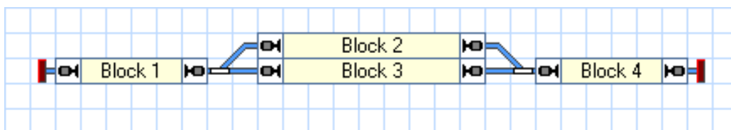
Abbildung 21: Komplettes Gleisbild mit Blocksymbolen
